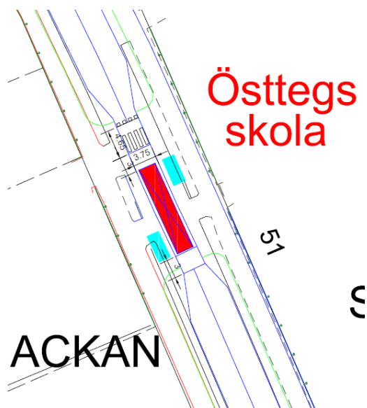
Figur 8-18 Förslag på utformning av hållplatsen vid Östtegs skola med timglashållplats.
