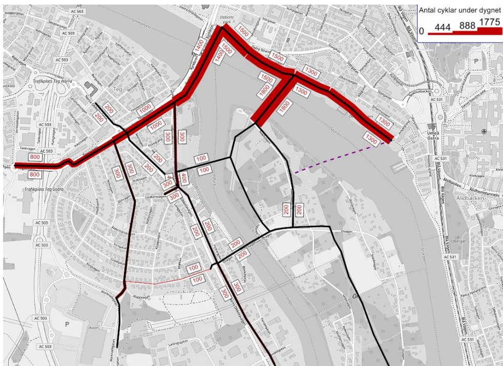
Figur 0-6 Cykelresor till och från Norra Ön år 2030 i scenario 1. Flödena i figuren visar endast cykelresor till/från Norra Ön samt de relationer där cykelmätningar finns idag vilket gör att figuren inte ger en heltäckande bild av cykelflödena som helhet. De cykelflöden som inkluderas i modellen utgår ifrån centrum med mätpunkter i Östteg, Universitetet, IKEA Avion och Röback
