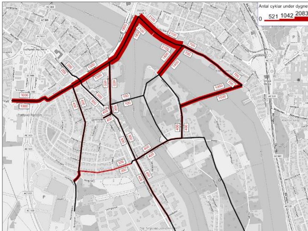
Figur 5-4 Cykelresor enligt scenario 2 när Norra Ön är fullt utbyggt, med den extra gång- och cykelbron mot universitetet. Flödena i figuren visar endast cykelresor till/från Norra Ön samt de relationer där cykelmätningar finns idag vilket gör att figuren inte ger en heltäckande bild av cykelflödena som helhet. De cykelflöden som inkluderas i modellen utgår ifrån centrum med målpunkter på Östteg, Universitetet, IKEA Avion och Röbbäck.
