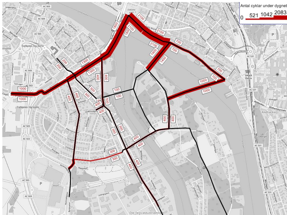
Figur 0-13 Cykelresor till och från Norra Örn år 2030 i scenario 2 med extra gång- och cykelbro. Flödena i figuren visar endast cykelresor till/från Norra Örn samt de relationer där cykelmätningar finns idag vilket gör att figuren inte ger en heltäckande bild av cykelflödena som helhet. De cykelflödena som inkluderas i modellen utgår ifrån centrum med målpunkter i Östteg, Universitetet, IKEA Avion och Röbbäck
