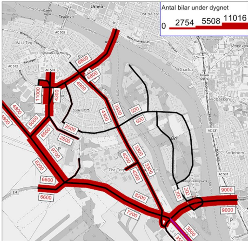
Figur 0-1 Dagens motorfordonsflöden i VISUM modell.
