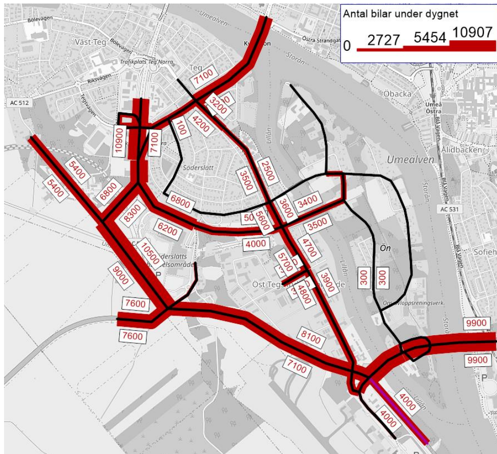
Figur 8-8 Prognostiserade motorfordonsflöden scenario 2 år 2040 med exploatering av Norra Ön och med Söderslättsvägen. I flödeskartan ingår ej alstrad trafik från Södra Ön utan redovisas separat i kapitel 8.6. Belastning på Skiljevägen fördelas mer troligt upp mellan Skiljevägen och Övägen vilket ej fångas upp av modellen för både nuläget och 2040.
