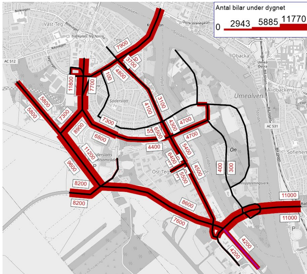
Figur 0-3 Prognostiserade motorfordonsflöden scenario 1 år 2040 med exploatering av Norra Ön och med Söderslättsvägen. I flödeskartan ingår ej alstrad trafik från Södra Ön utan redovisas separat i kapitel 8.6. Belastning på Skiljevägen fördelas mer troligt upp mellan Skiljevägen och Övägen vilket ej fångas upp av modellen för både nuläget och 2040.
