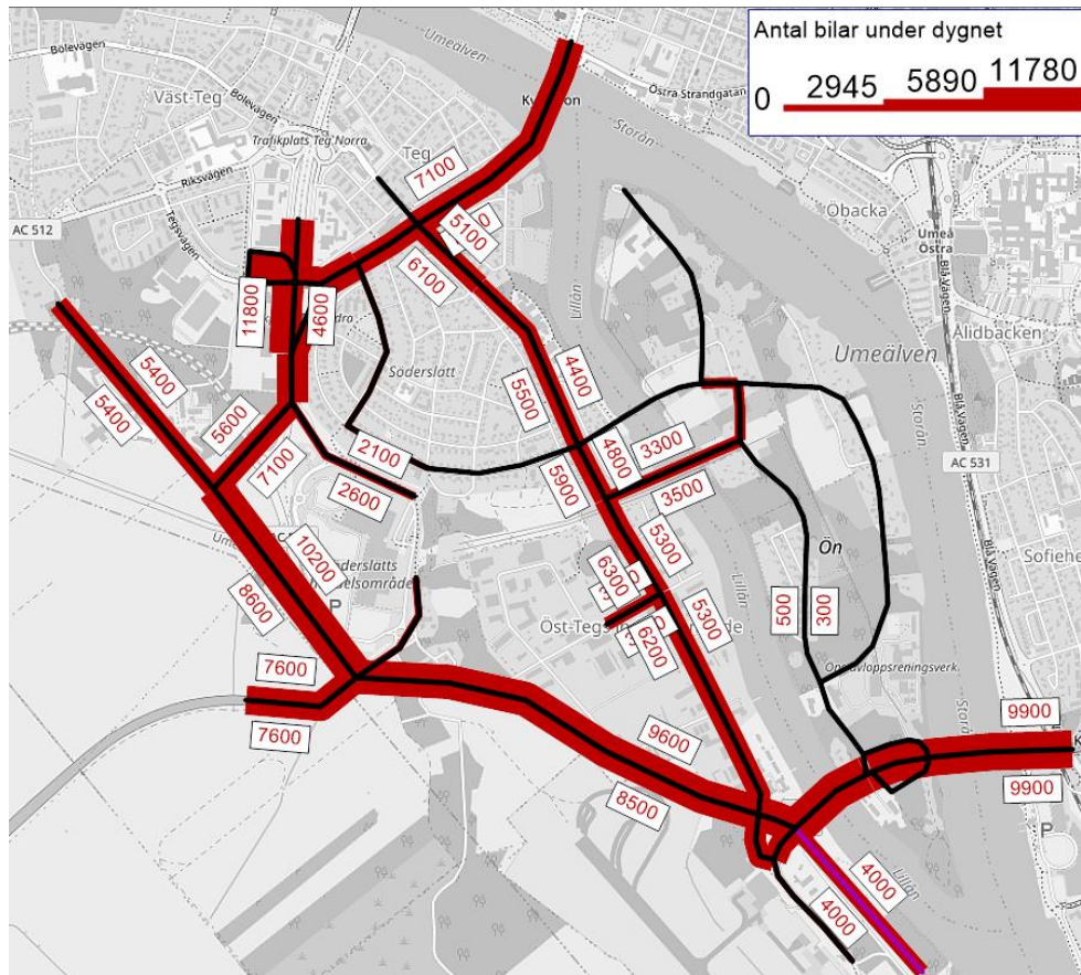
Figur 0-10 Prognostiserade motorfordonsflöden scenario 2 år 2040 med exploatering av Norra Ön och utan Söderslättsvägen.
