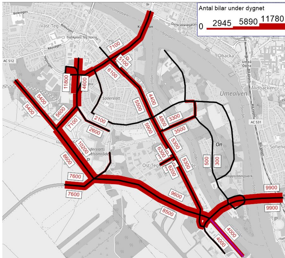
Figur 8-7 Prognostiserade motorfordonsflöden scenario 2 år 2040 med exploatering av Norra Ön och utan Söderslättsvägen. I flödeskartan ingår ej alstrad trafik från Södra Ön utan redovisas separat i kapitel 8.6. Belastning på Skiljevägen fördelas mer troligt upp mellan Skiljevägen och Övägen vilket ej fångas upp av modellen för både nuläget och 2040.
