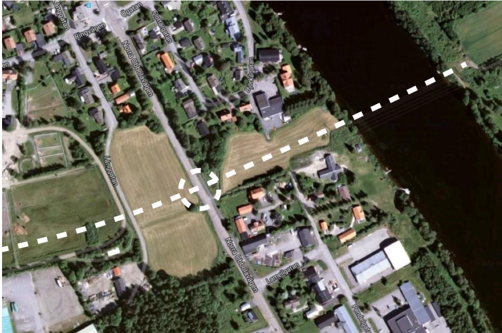
Figur 0-3 Framtida cirkulation Norra Obbolavägen – Söderslättsvägen/ nya bron från ön.
