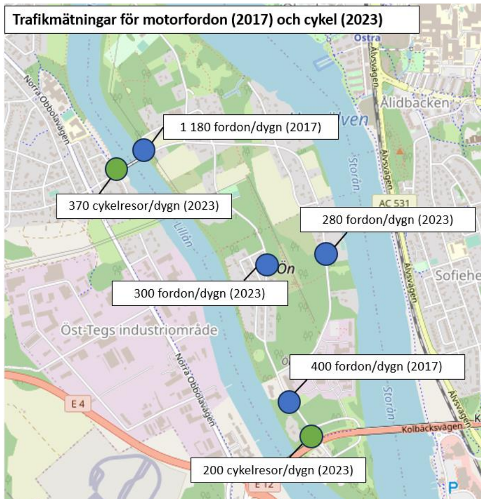
Figur 0-2 Trafikmätningar för motorfordonstrafik (2017/2023) samt cykeltrafik (2023).
