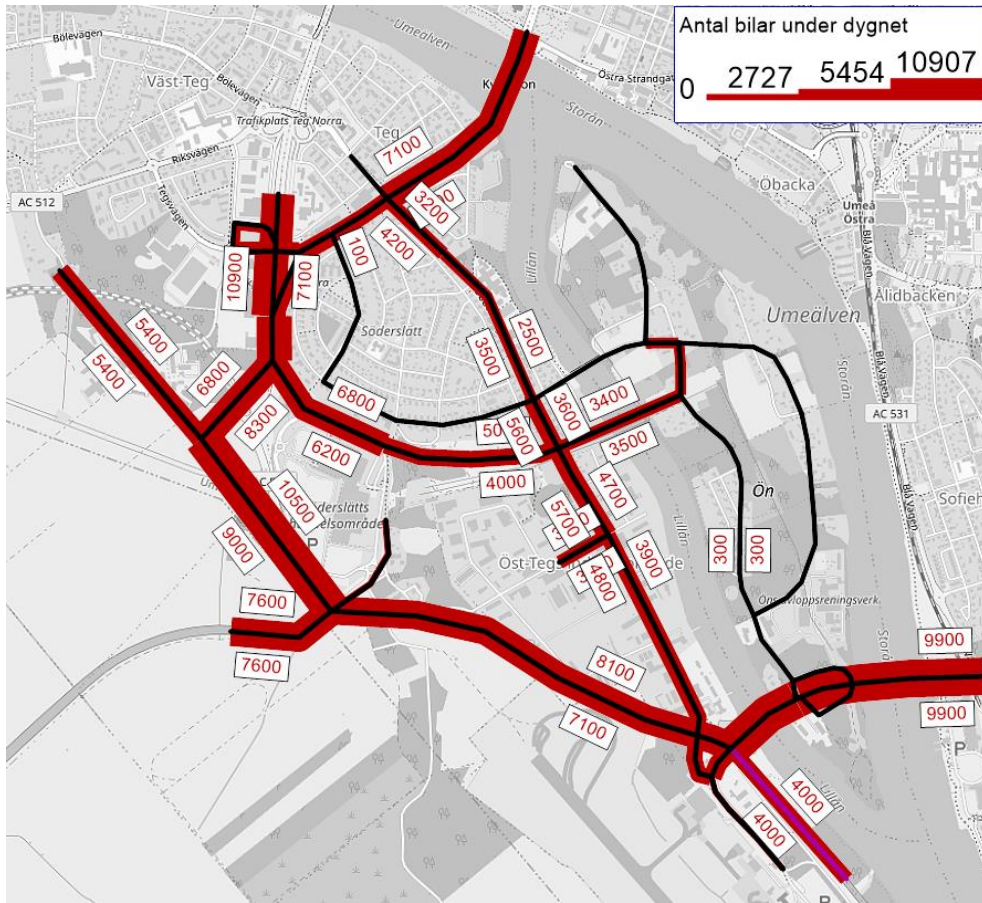
Figur 0-11 Prognostiserade motorfordonsflöden scenario 2 år 2040 med exploatering av Norra Ön och med Söderslättsvägen.
