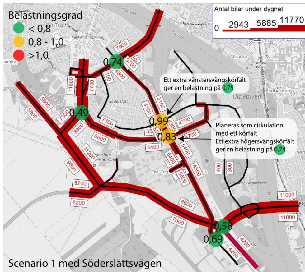
Figur 8-9 Kapacitet i korsningspunkter med trafikflöden enligt scenario 1 och med förutsättning att Söderslättsvägen byggs ut. Belastningsgraden visas för den tillfart som har högst belastningsgrad i varje korsningspunkt.
