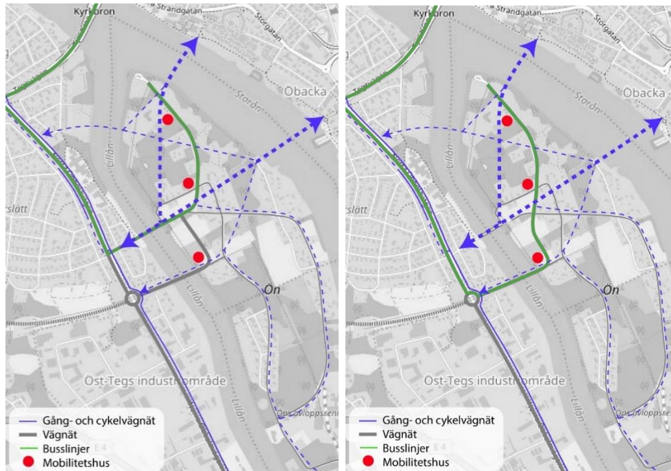
Figur 0-1 Två alternativa strukturer för trafiken på Norra Ön. Båda alternativen prioriterar gång och cykel. Det som framför allt skiljer dem åt är vilken bro som används för busstrafiken, vilket i sin tur påverkar gatustrukturen. Blå streckade linjer visar vilka samband som är viktiga att stärka för gång och cykel, och är utgångspunkt för mer detaljerade lösningar.
