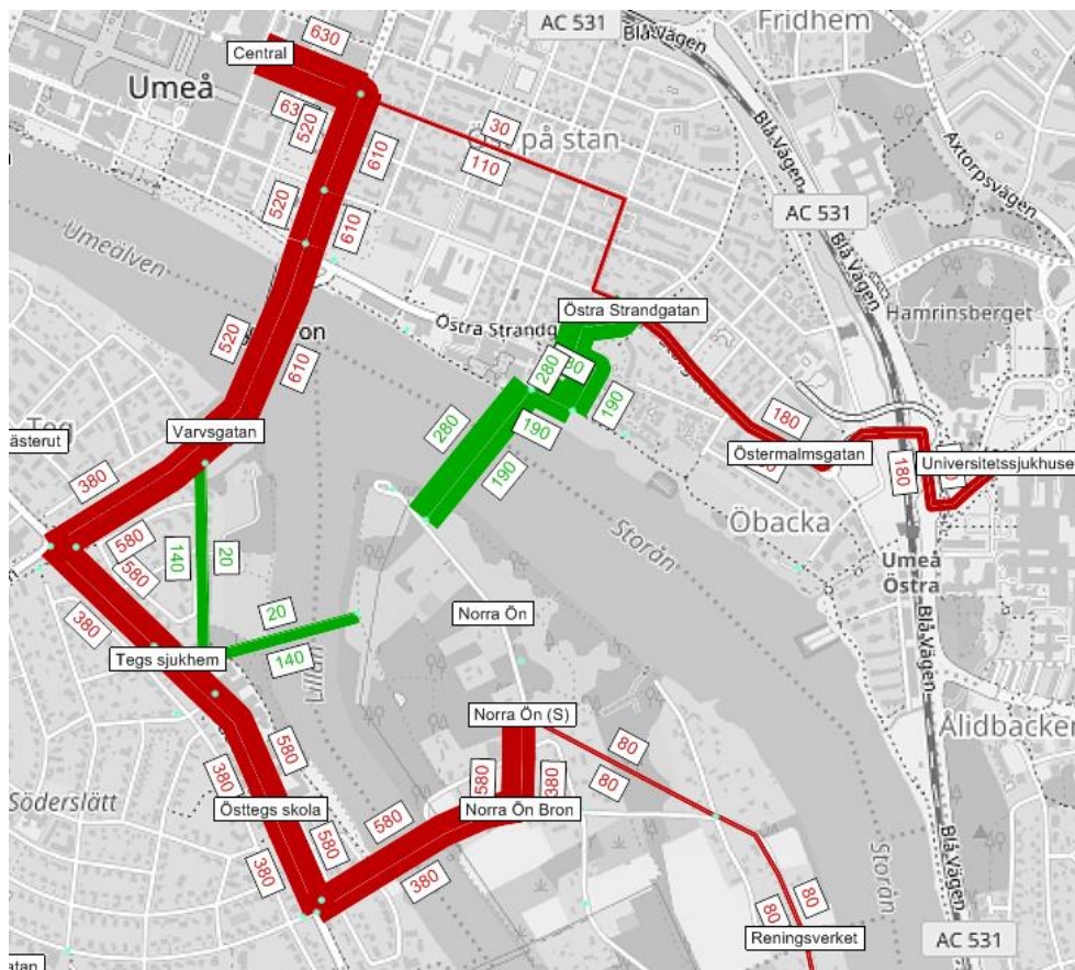
Figur 6-9 Alternativ 2: Med målstyrd planering kan Norra Öns exploatering ge ovanstående belastning på busstråken per vardagsdygn (röd). Kollektivtrafikresenärer som går till hållplats utanför Norra Ön (grön).
