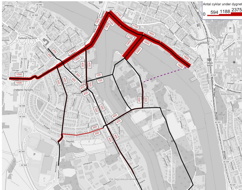
Figur 0-12 Cykelresor till och från Norra Ön år 2030 i scenario 2. Flödena i figuren visar endast cykelresor till/från Norra Ön samt de relationer där cykelmätningar finns idag vilket gör att figuren inte ger en heltäckande bild av cykelflödena som helhet. De cykelflöden som inkluderas i modellen utgår ifrån centrum med målpunkter i Östteg, Universitetet, IKEA Avion och Röbäck
