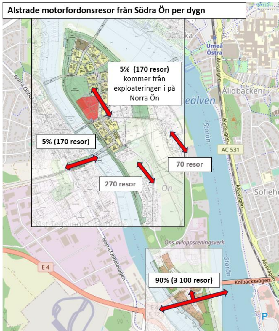
Figur 0-3 Fördelning av alstrade motorfordonsresor från Södra Ön per dygn
