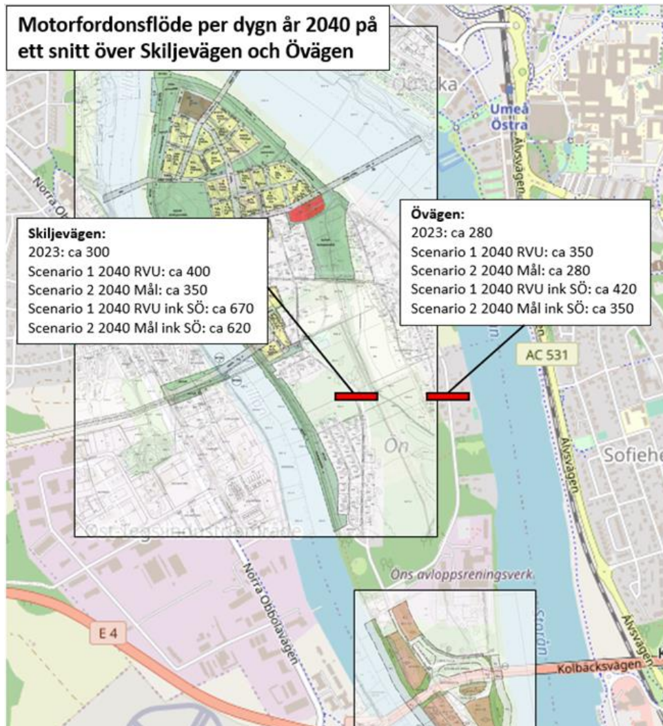
Figur 0-4 Motorfordonsflöde på Skiljevägen och Övägen för nuläget samt prognosår 2040 utifrån givna förutsättningar.
