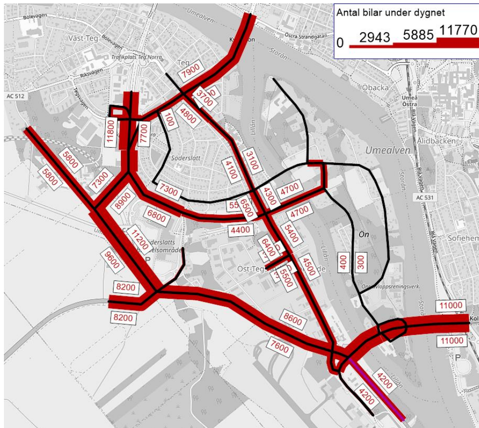
Figur 8-6 Prognostiserade motorfordonsflöden scenario 1 år 2040 med exploatering av Norra Ön och med Söderslättsvägen. I flödeskartan ingår ej alstrad trafik från Södra Ön utan redovisas separat i kapitel 8.6. Belastning på Skiljevägen fördelas mer troligt upp mellan Skiljevägen och Övägen vilket ej fångas upp av modellen för både nuläget och 2040.
