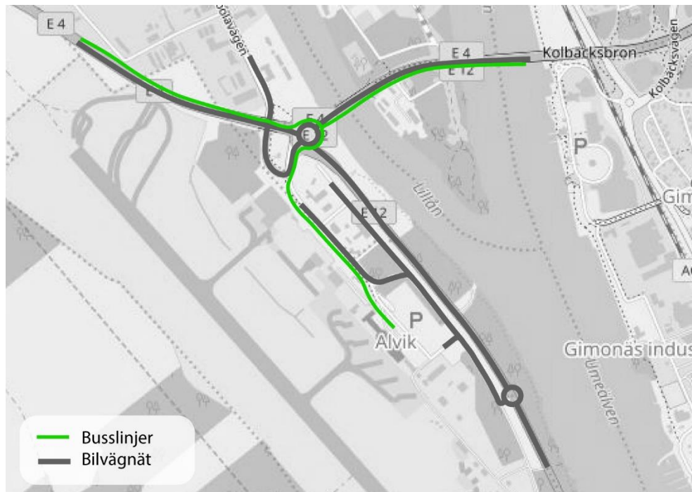
Figur 8-22 En ny infart till flygplatsen skulle avlasta korsningen Flygplatsvägen-Norra Obbolavägen.
