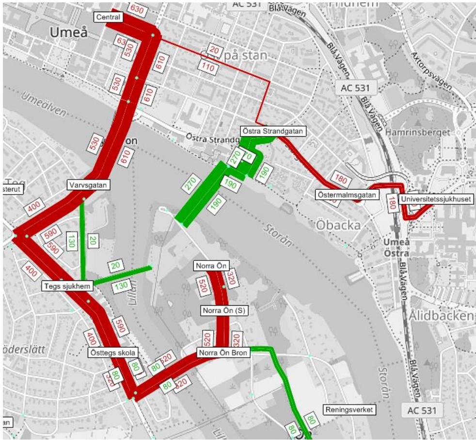
Figur 6-7 Alternativ 1: Med målstyrd planering kan Norra Öns exploatering ge ovanstående belastning på busstråken per vardagsdygn (röd). Kollektivtrafikresenärer som går till hållplats utanför Norra Ön (grön).
