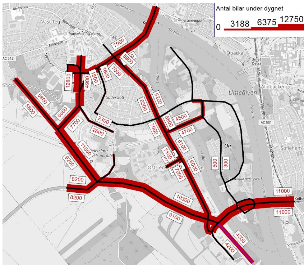
Figur 0-2 Prognostiserade motorfordonsflöden scenario 1 år 2040 med exploatering av Norra Ön och utan Söderslättsvägen. I flödeskartan ingår ej alstrad trafik från Södra Ön utan redovisas separat i kapitel 8.6. Belastning på Skiljevägen fördelas mer troligt upp mellan Skiljevägen och Övägen vilket ej fångas upp av modellen för både nuläget och 2040.
