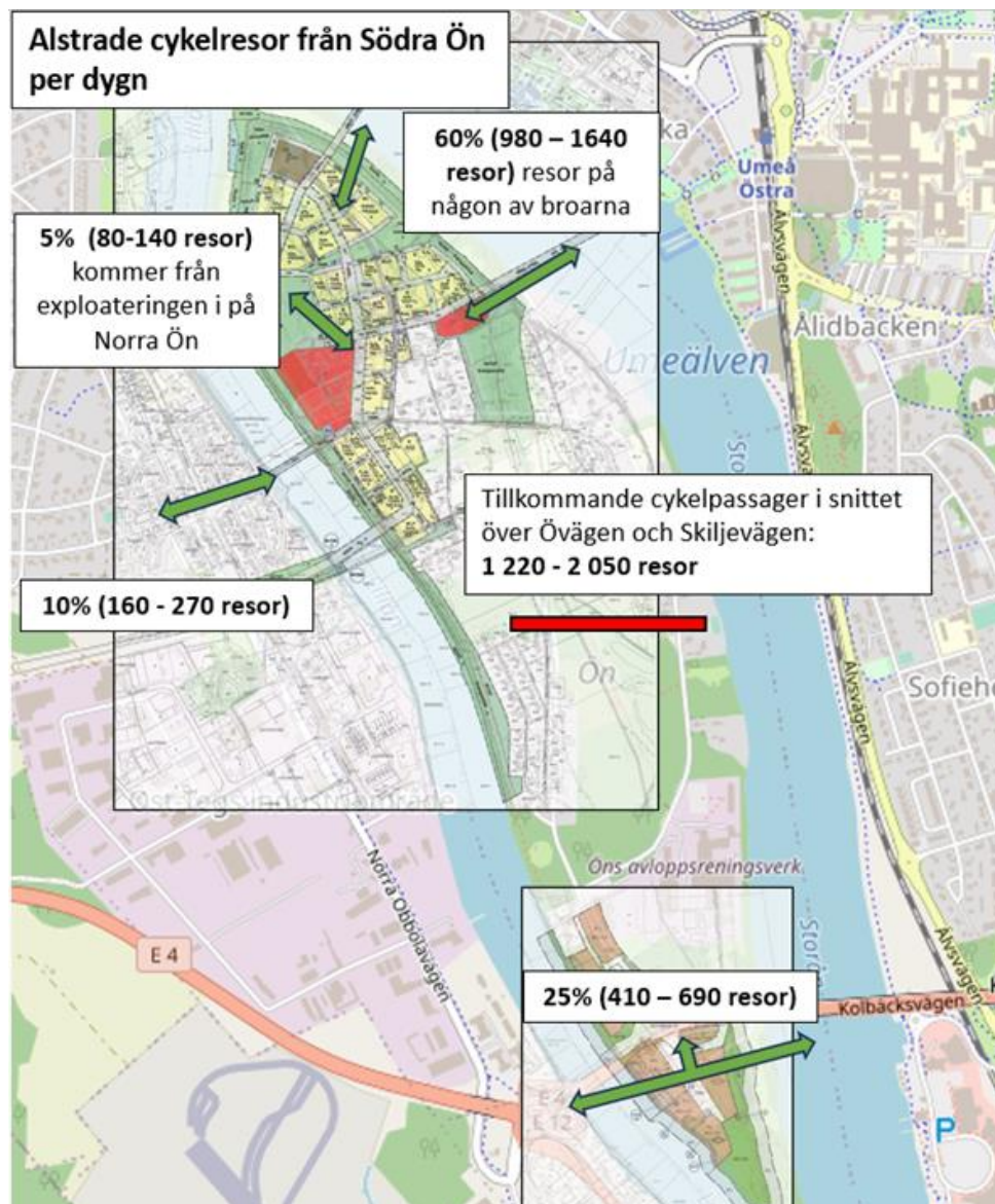
Figur 0-5 Antal alstrade cykelresor från exploateringen av Södra Ön. Rött snitt markerar tillkommande flöde fördelat på Skiljevägen och Övägen.
