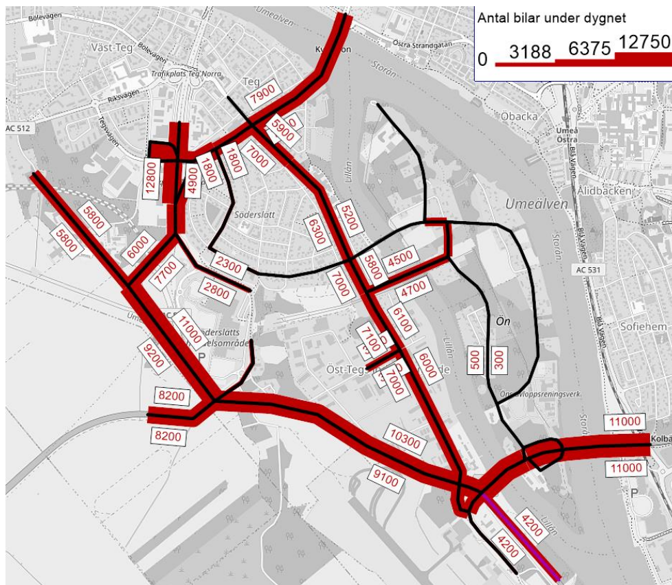
Figur 8-5 Prognostiserade motorfordonsflöden scenario 1 år 2040 med exploatering av Norra Ön och utan Söderslättsvägen. I flödeskartan ingår ej alstrad trafik från Södra Ön utan redovisas separat i kapitel 8.6. Belastning på Skiljevägen fördelas mer troligt upp mellan Skiljevägen och Övägen vilket ej fångas upp av modellen för både nuläget och 2040.
