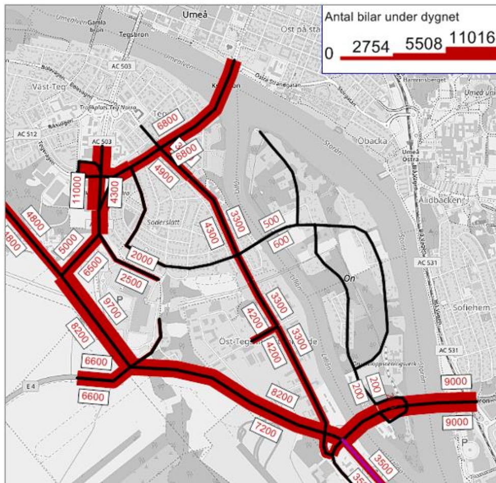
Figur 8-3 Dagens (2017) motorfordonsflöden i kalibrerad simuleringsmodell (Visum).
